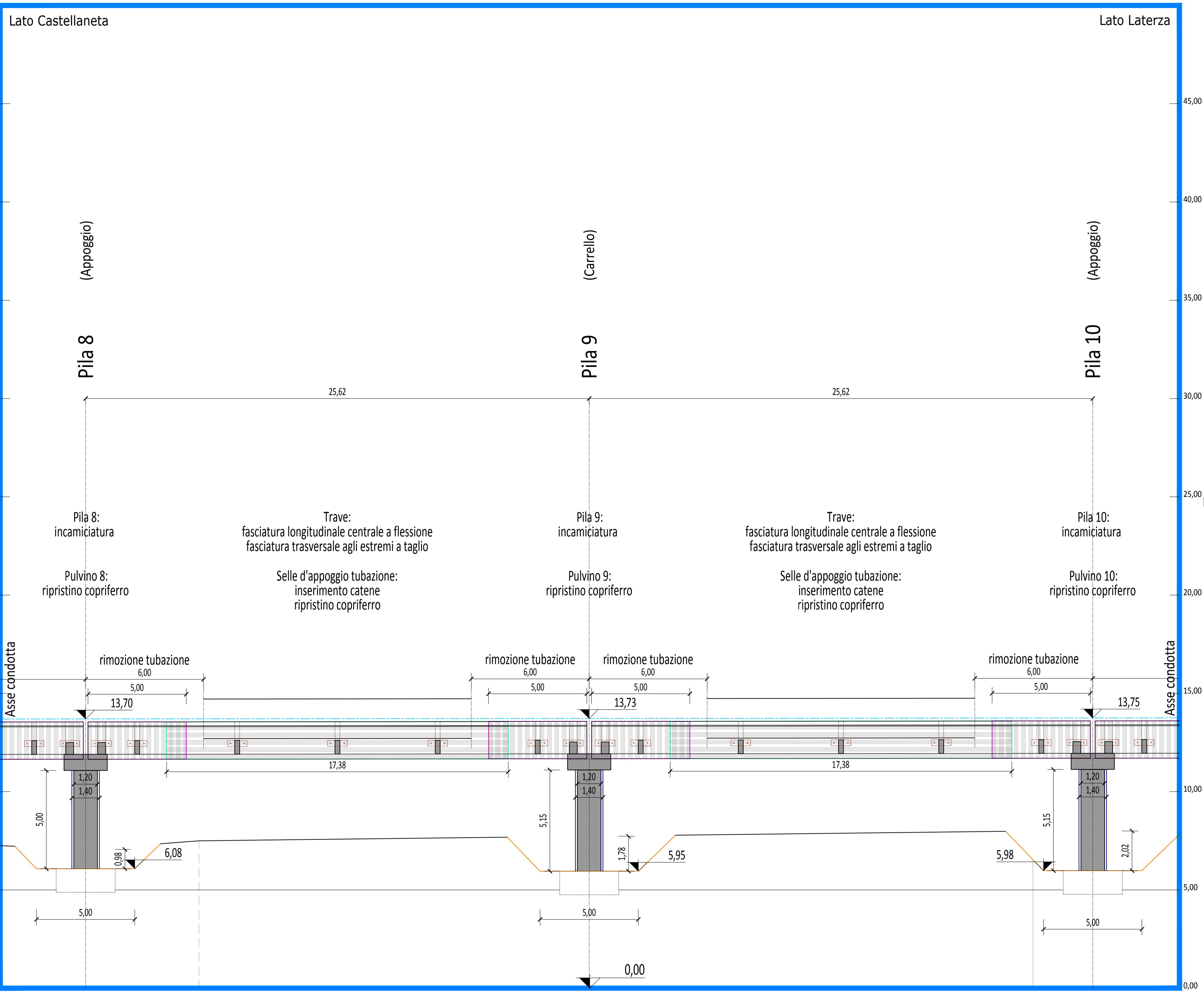
Profilo longitudinale dalla Pila 8 alla Pila 10
